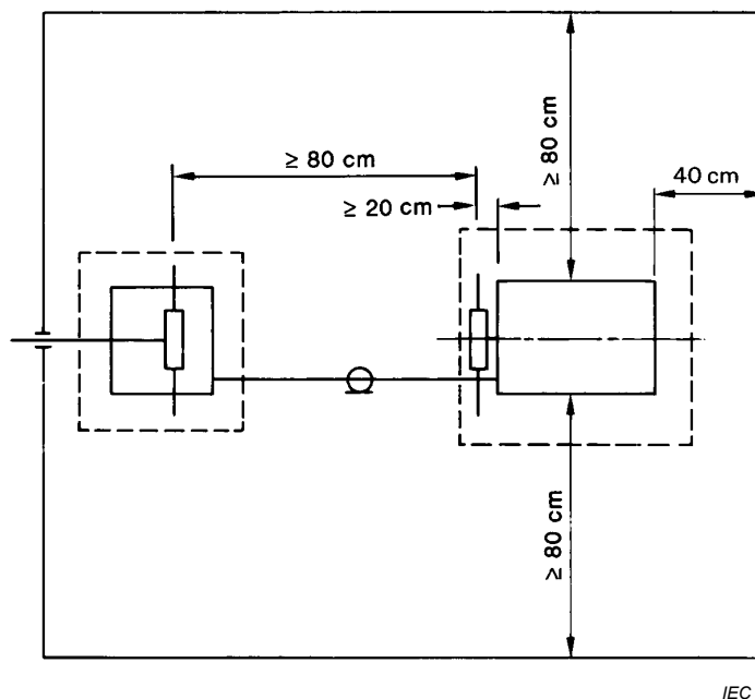
Figure 6 – Mesure de la tension perturbatrice à fréquence radioélectrique injectée dans le réseau électrique (vue de dessus) (voir 5.3.1)
