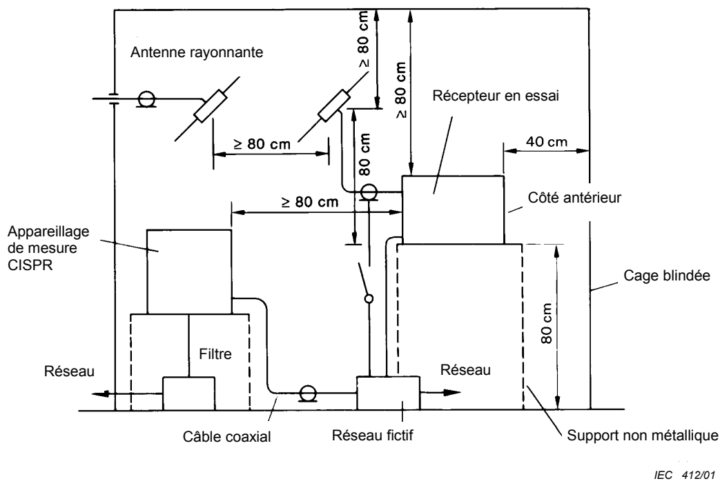
Figure 5 – Mesure de la tension perturbatrice à fréquence radioélectrique injectée dans le réseau électrique (voir 5.3.1)
